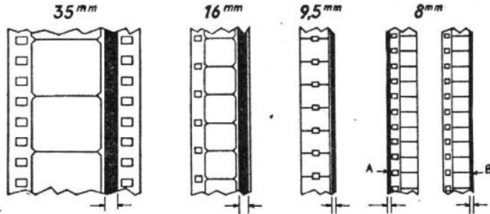
FIG. 3. — Dispositions et largeurs comparées des pistes magnétiques sur les différents formats
