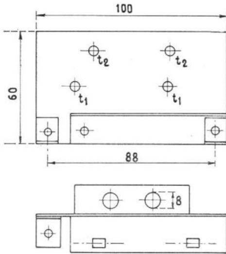
Fig. 4. — Le radiateur des transistors de sortie
