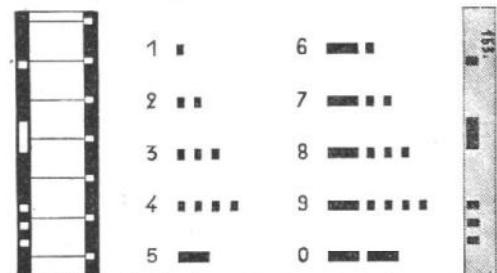
FIG. 4. — Code de marquage pour la synchronisation optique entre le film muet et la bande magnétique (Auto Script Martin)
