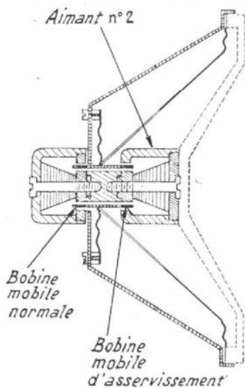
FIG. 4. — Coupe du haut-parleur Gego avec bobine mobile normale et bobine mobile d'asservissement
