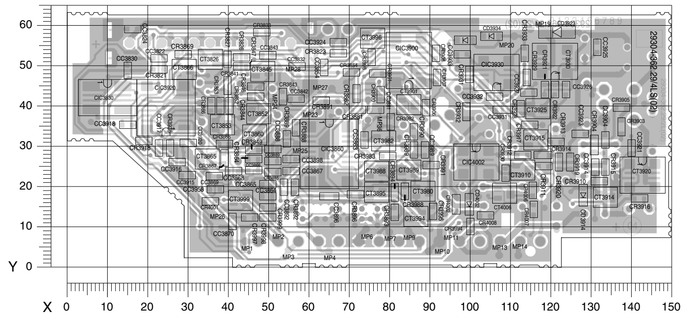
Côte soudures, Vue de dessous / Solder Side, Bottom View
