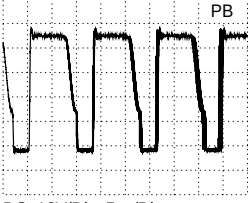
DC, 10V/Div, 5µs/Div Trafo 5330-(4), 5331-(4) 50
