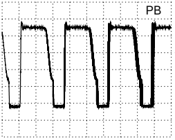
DC, 10V/Div, 5µs/Div Trafo 5330-(4), 5331-(4) 50
