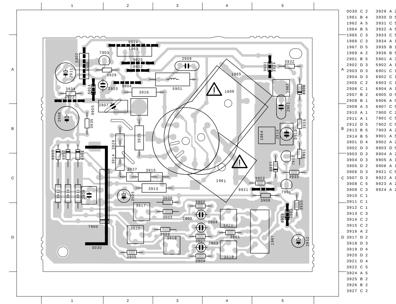
Vue côté composants / View of Component Side
